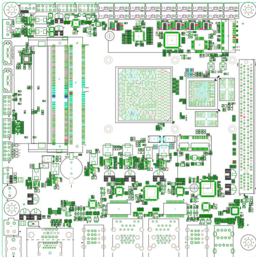
正面布局图
