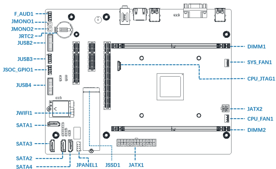
接口位置图
